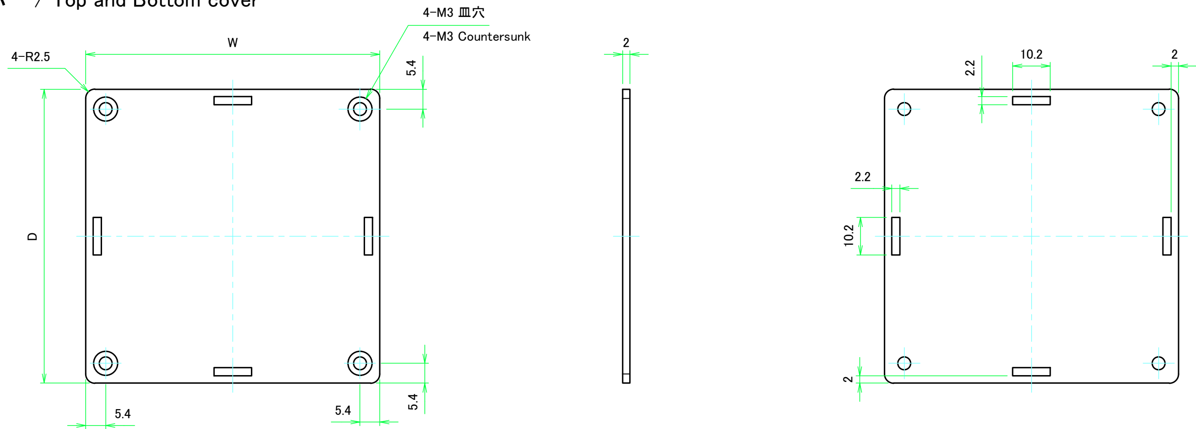
上カバー裏面 / Top cover Backside
